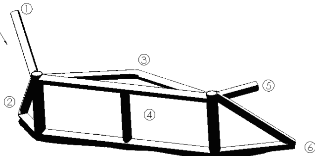
ESQUEMA 3D PROTECCION INTERNA PONTON - TC 4000 CORDOBES
