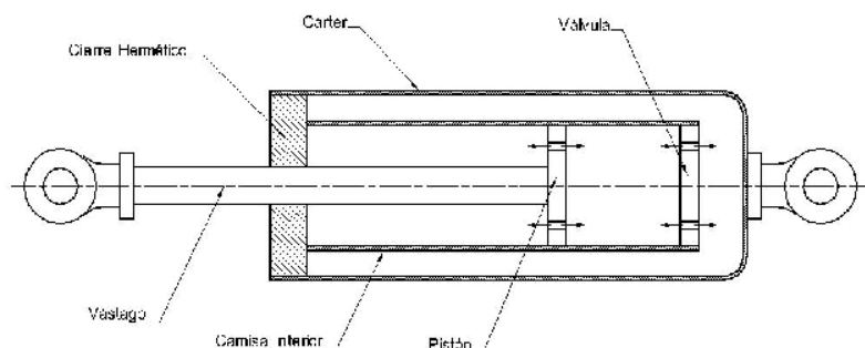
Esquema del amortiguador
